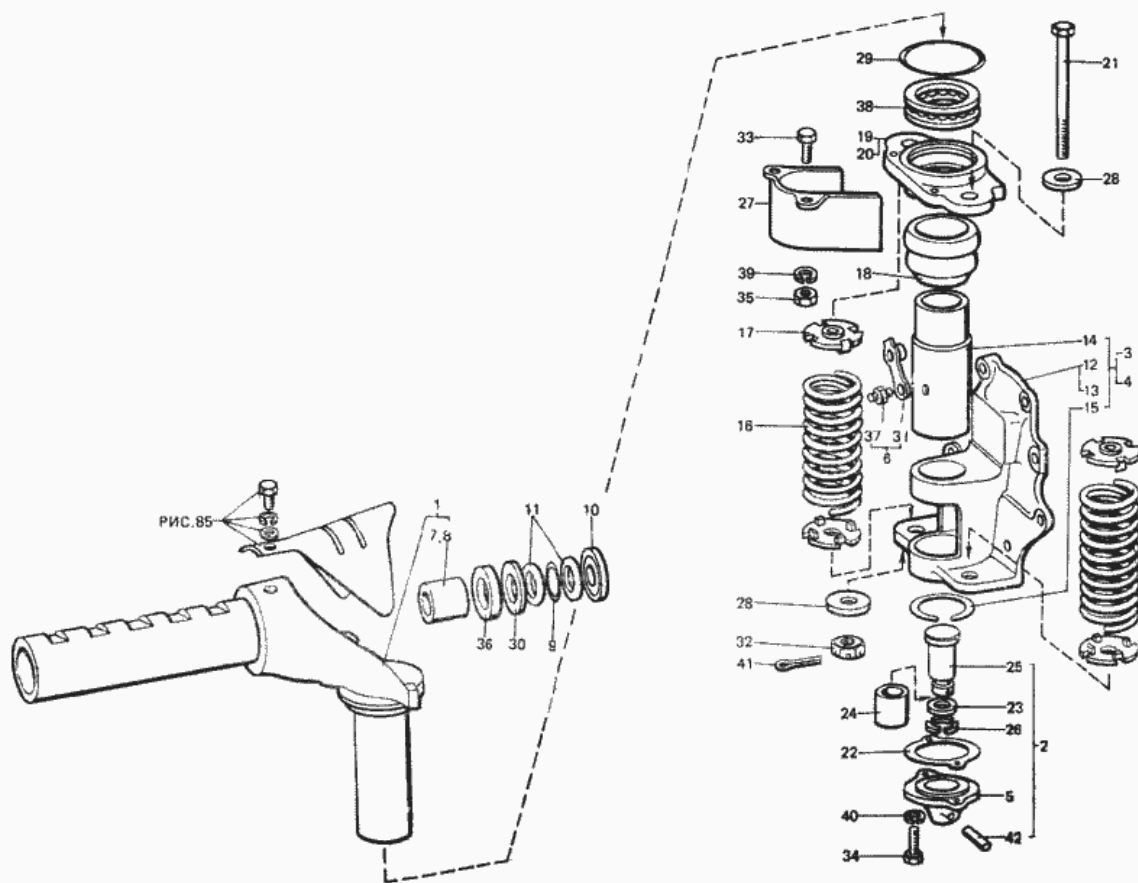
Рис. 89. Подвеска колеса Т40А-2305010-А, Т40АН-2305010-А
